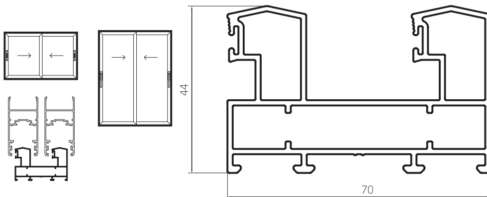
Marco Dos Hojas Corredizas 1,405 kg/m 08011 Barras de 6.05m
