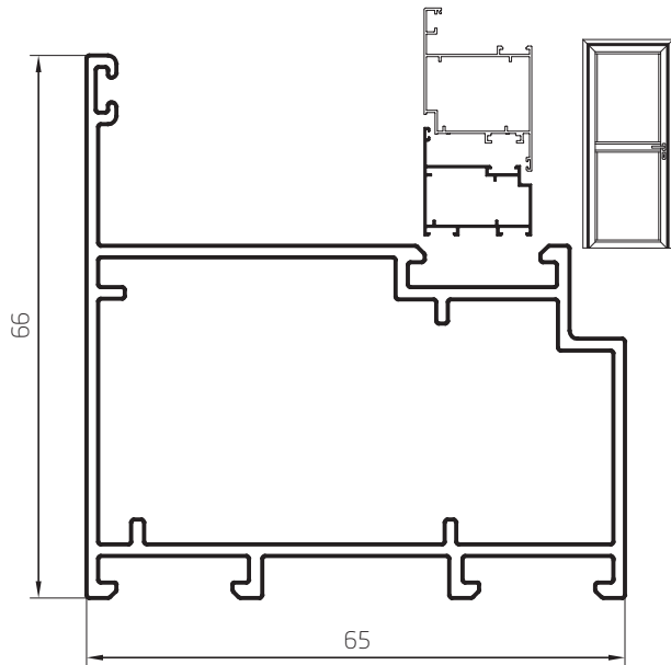
Marco Puerta de Abrir 1,106 Kg/m 08102 Barras de 6.20m
