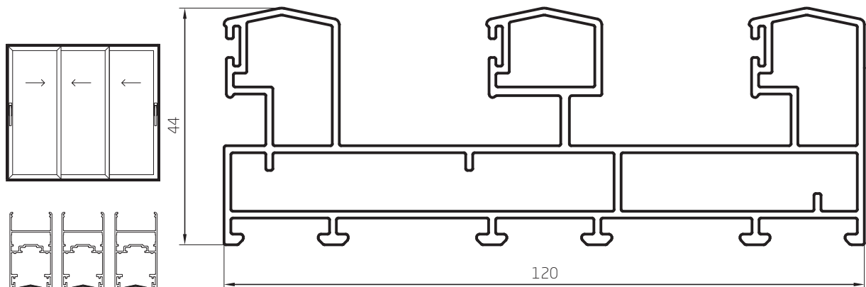
Marco Ventana Corrediza 2,127 Kg/m 08001 Barras de 6.05m
