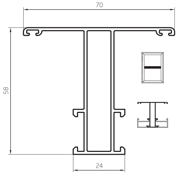
Travesaño 0,900 Kg/m 08204 Barras de 6.05m
