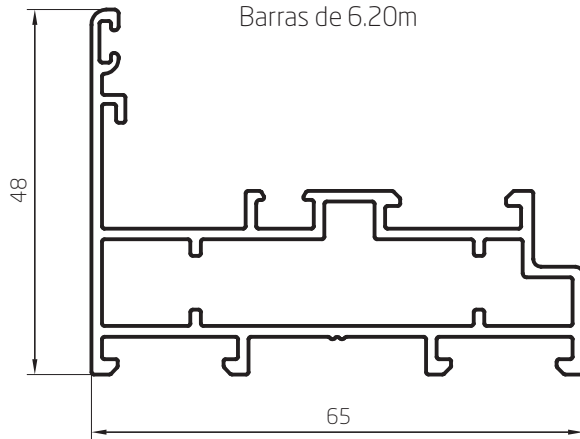
Marco Ventana de abrir 65mm 1,000 Kg/m 08018 Barras de 6.05m
