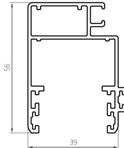
Mosquitero 0,980 Kg/m 08005 Barras de 6.05m
