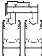
Premarco 0,360 Kg/m 08030 Barras de 6.05m
