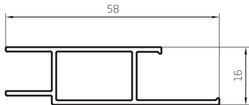
Premarco 0,425 Kg/m 08031 Barras de 6.05m
