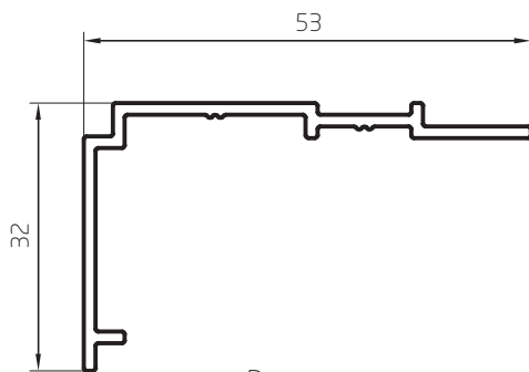
Premarco 0,360 Kg/m 08030 Barras de 6.05m
