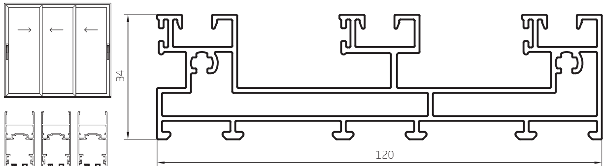
Marco Inferior Transitable 1,957 kg/m 08009 Barras de 6.05m
