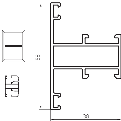
Travesaño Curvo 0,748 kg/m 03203 Barras de 6.05m 6 Barras por Paquete
