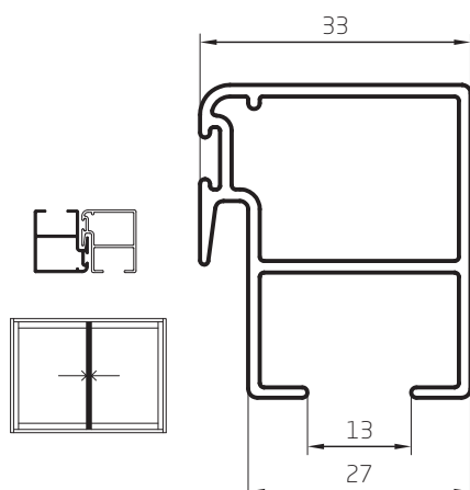
Parante Central 0,603 kg/m 03004 Barras de 6.05m 6 Barras por Paquete
