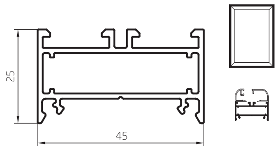
Marco Doble Contravidrio 0,652 kg/m 03202 Barras de 6.05m 6 Barras por Paquete
