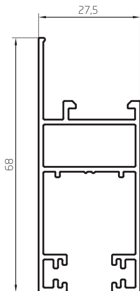
Hoja 68mm 45° con contravariado 0,795 kg/m 03314 Barras de 6.05m 6 Barras por Paquete
