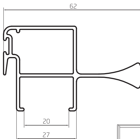
Parante Central Reforzado DVH 0,892 kg/m 03039 Barras de 6.05m 4 Barras por Paquete
