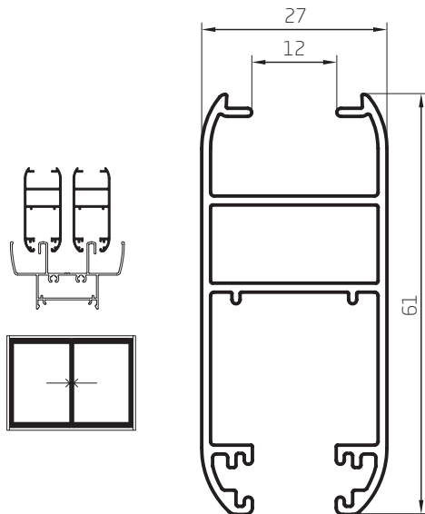
S Hoja 45° 0,765 kg/m 03014 Barras de 6.05m 6 Barras por Paquete
