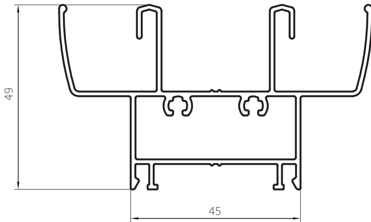
Marco Ventana Corrediza a 90° 1,140 kg/m 06401 Barras de 6.05m
