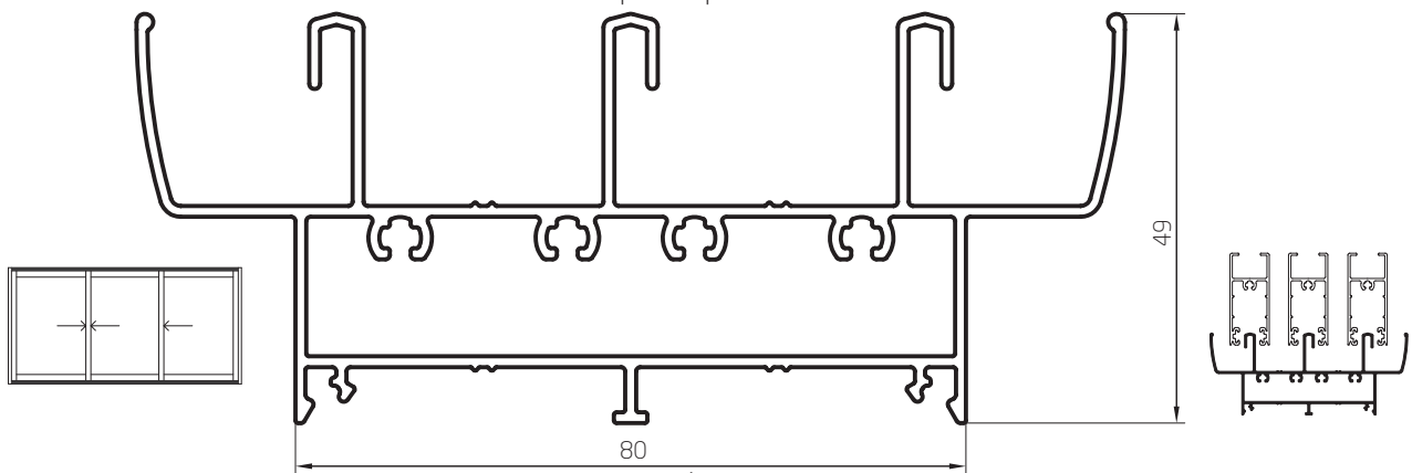
Marco 3 Guías 1,665 kg/m 03061 Barras de 6.05m 2 Barras por Paquete
