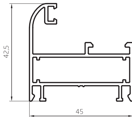
Marco Paño Fijo Curvo 0,767 kg/m 06421 Barras de 6.05m
