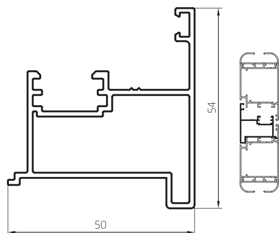
Encuentro Central 0,827kg/m 03105 Barras de 6.05m 6 Barras por Paquete
