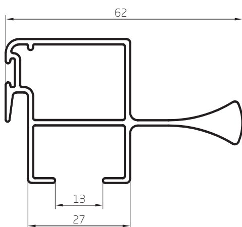
Parante Central Reforzado 0,916 kg/m 03009 Barras de 6.05m 4 Barras por Paquete
