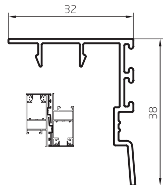
Encuentro Central Hoja 3314 0,317 kg/m 03313 Barras de 6.05m 20 Barras por Paquete
