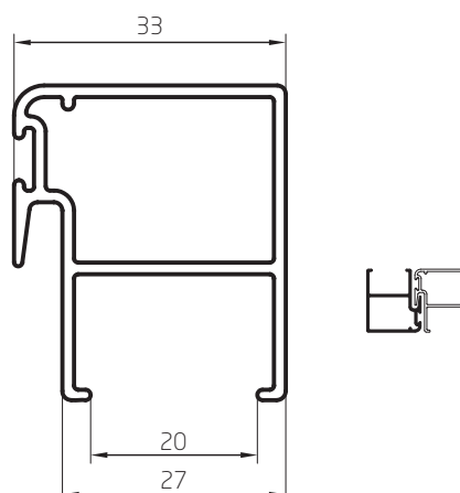
Parante Central DVH 0,577 kg/m 03034 Barras de 6.05m 6 Barras por Paquete
