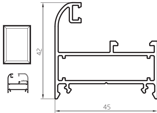
Marco Curvo 0,748 kg/m 03201 Barras de 6.05m 6 Barras por Paquete
