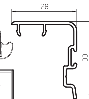
Encuentro Central 0,256 kg/m 03013 Barras de 6.05m 20 Barras por Paquete
