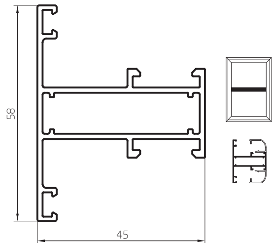
Travesaño Recto 0,797 kg/m 03204 Barras de 6.05m 6 Barras por Paquete
