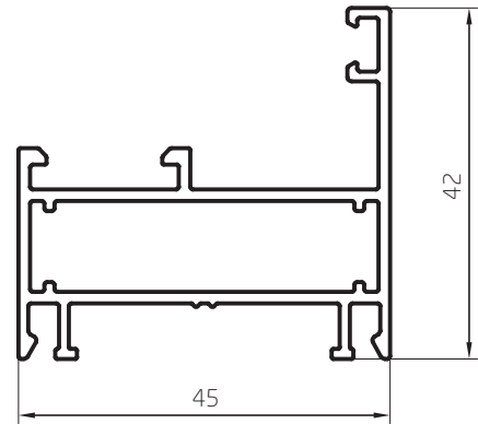
Marco Puerta 0,728 kg/m 06402 Barras de 6.20m
