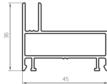
Jamba Ventana Corrediza a 90° 0,615 kg/m 06410 Barras de 6.05m
