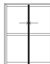
Parante Central Reforzado DVH 0,892 kg/m 03039 Barras de 6.05m 4 Barras por Paquete
